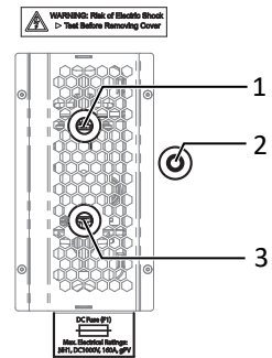
Abb. 49: Spannungsfreiheit sicherstellen
