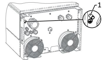
Abb. 24: Zusätzlicher Erdungspunkt
