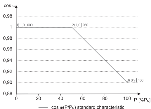
Abb. 34: \cos \varphi / (P/P_n) Standard Kennlinie mit 3 Stützstellen
