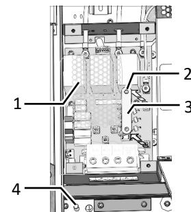
Abb. 16: 5-Leiter Anschluss
