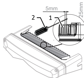
Abb. 52: Kühlrippen reinigen
