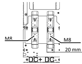
Abb. 23: DC-Anschluss B-Version
