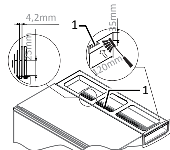
Abb. 51: Kühlrippen reinigen
