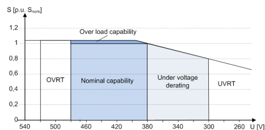
Abb. 33: Netzspannungsabhängige Scheinleistung für Speichergeräte mit U_N 220/380, 230/400, 240/415V
