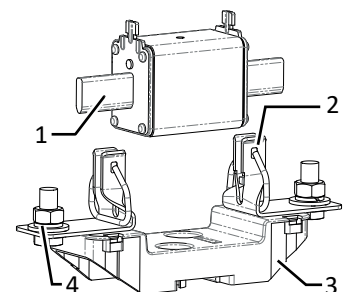
Abb. 55: DC-Sicherung einlegen
