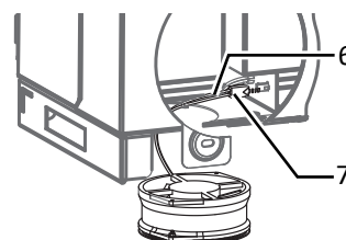
Abb. 54: Lüfterstecker abziehen
