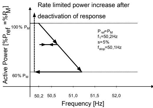
Abb. 42: Beispielverhalten mit Hysterese (Modus 1)
