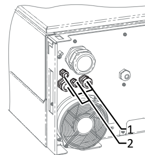
Abb. 26: Ethernet-Leitung einführen
