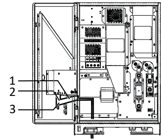
Abb. 27: Leitungen für Schnittstellen verlegen
