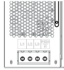
Abb. 18: 4-Leiter_Anschluss
