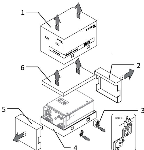
Abb. 9: Kartonage öffnen
