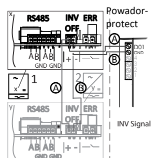
Abb. 30: Gerät mit Powador-protect verbinden
