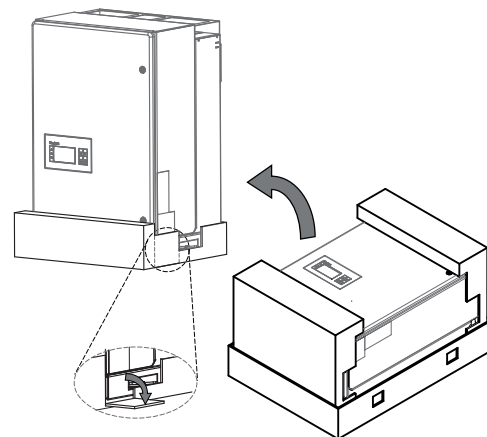
Abb. 10: Gerät aufrichten
