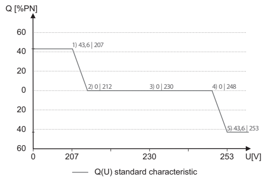
Abb. 35: Q(U) Standard Kennlinie mit 5 Stützstellen
