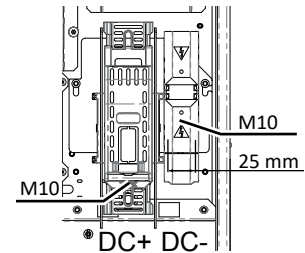
Abb. 22: DC_Anschluss M-Version
