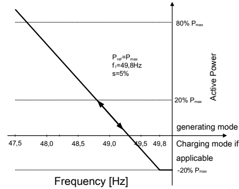
Abb. 43: Beispielverhalten ohne Hysterese (Modus 2) Zum Zeitpunkt der Aktivierung befindet sich der Wechselrichter im Ladebetrieb mit 20 % Ladeleistung.
