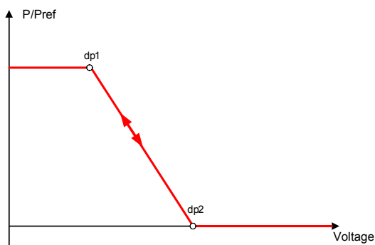
Abb. 36: Beispiel-Kennlinie ohne Hysterese
