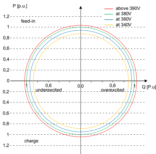
Abb. 32: P-Q Betriebsbereich für Speichergeräte mit U_N 220/380V, 230/400V, 240/415V ( Q_{max}=S_{max} )
