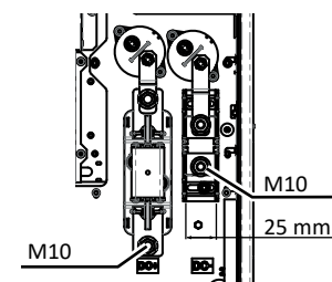
Abb. 21: DC-Anschluss XL-Version
