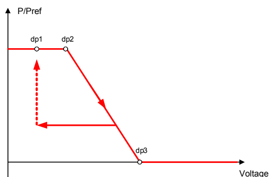
Abb. 37: Beispiel-Kennlinie mit Hysterese und einer Deaktivierungsschwelle unterhalb der Aktivierungsschwelle
