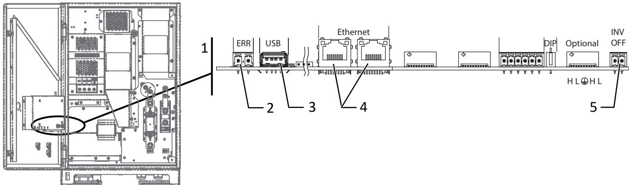
Abb. 25: Kommunikationsplatine: Anschluss und Belegung der Schnittstellen
