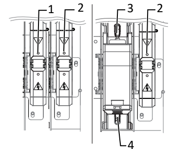
Abb. 50: Spannungsfreiheit sicherstellen: Basic, M-Version
