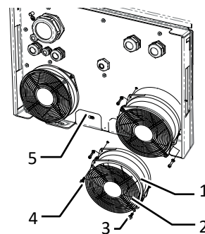
Abb. 53: Lüfter demontieren
