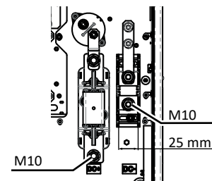
Abb. 20: DC-Anschluss L-Version
