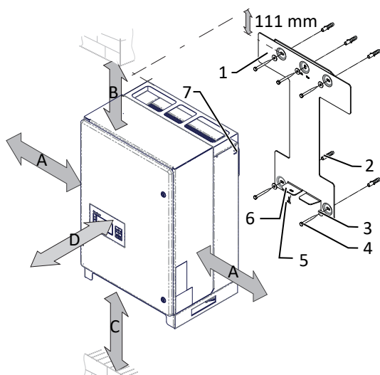
Abb. 11: Mindestabstände für Wandmontage
