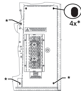
Abb. 19: Schutzabdeckung entfernen
